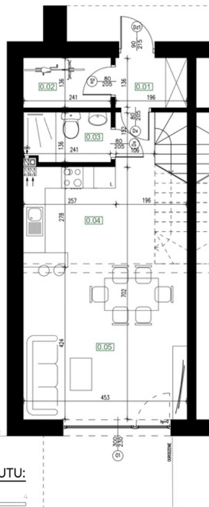
RZUT PARTERU |
